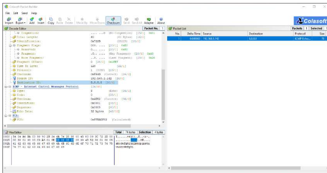
Рисунок 19 – Окно Packet Builder
