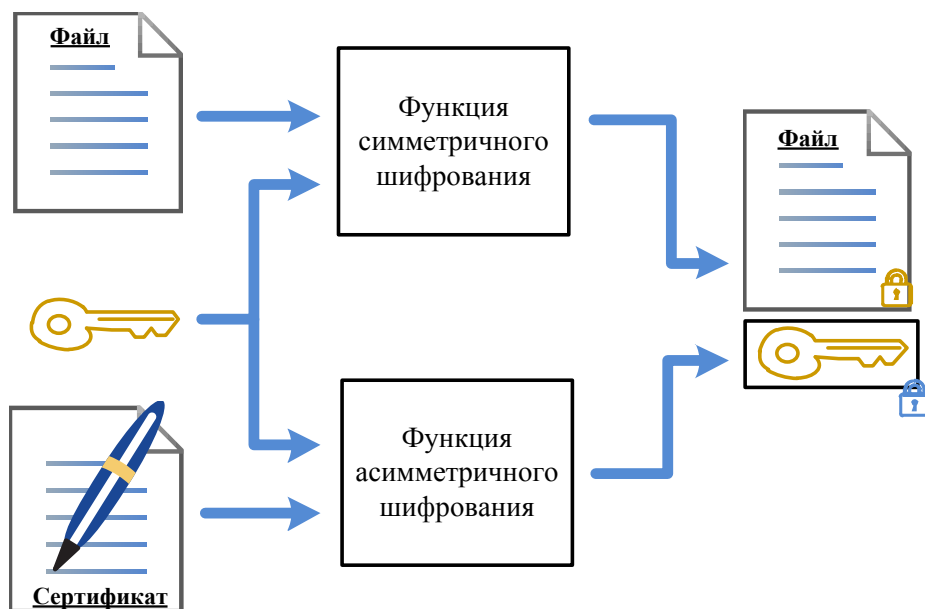
Рис. 1.1. Схема зашифрования файла
