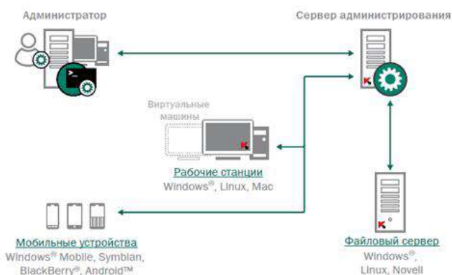
Рисунок 1 – Логика использования Kaspersky Security Center при защите сети организации.
