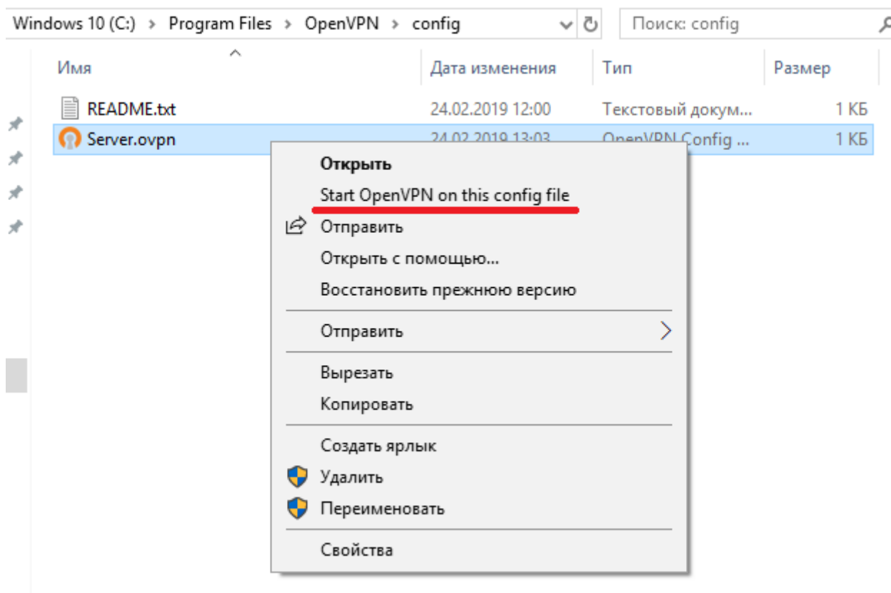
Рисунок 4.3 – Запуск сервера
