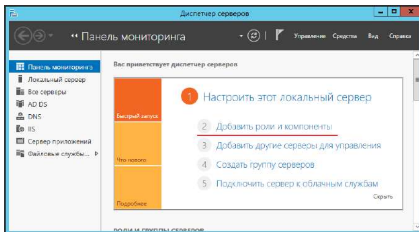
Рис. 2. Диспетчер серверов
