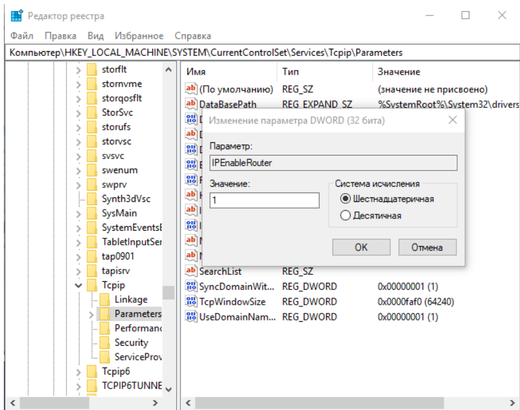
Рисунок 4.1 – Редактор реестра
