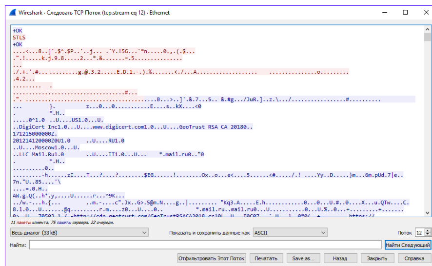
Рисунок 15 – Перехваченный поток
