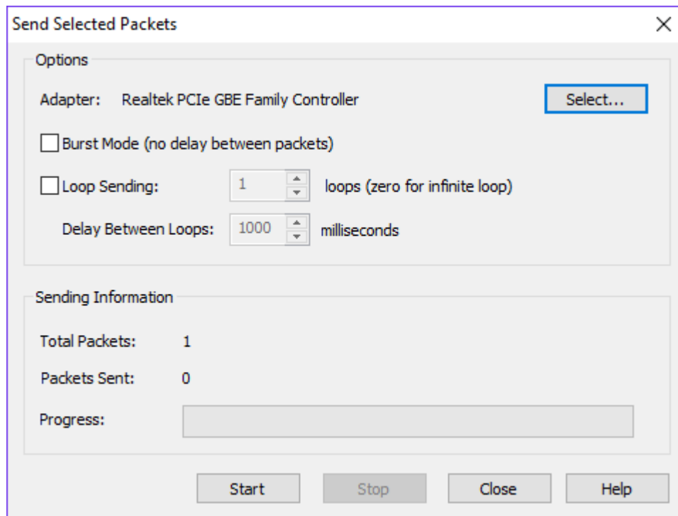
Рисунок 19 – Отправка пакета
