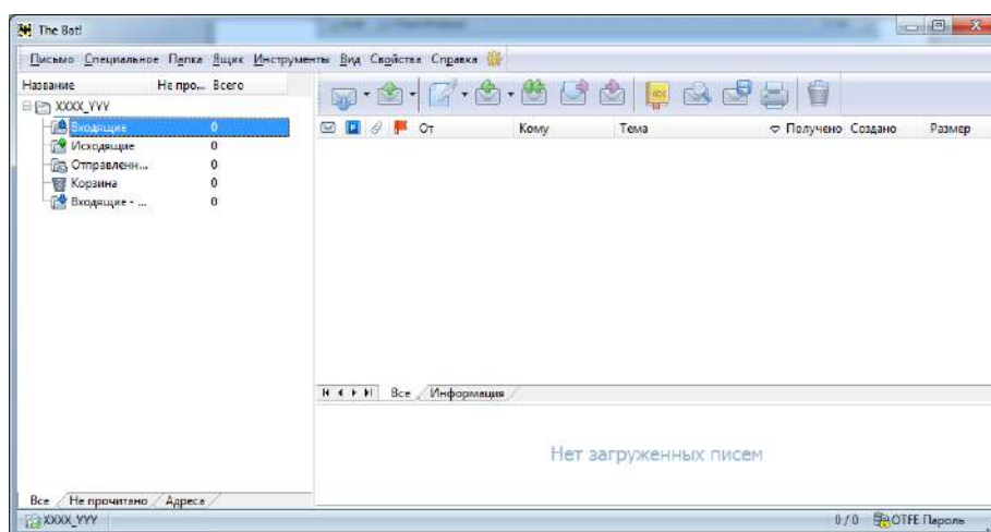
Рис.11 – Интерфейс программы
