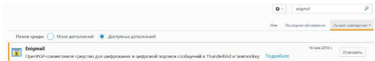
Рис. 4 поиск Enigmail
