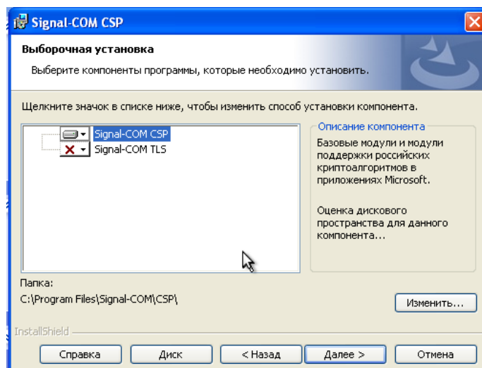
Рисунок 4.3 — Выбор компонентов
