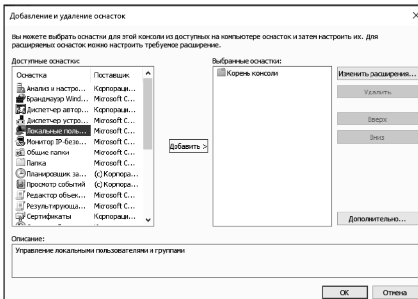
Рис. 6. Добавление оснастки
