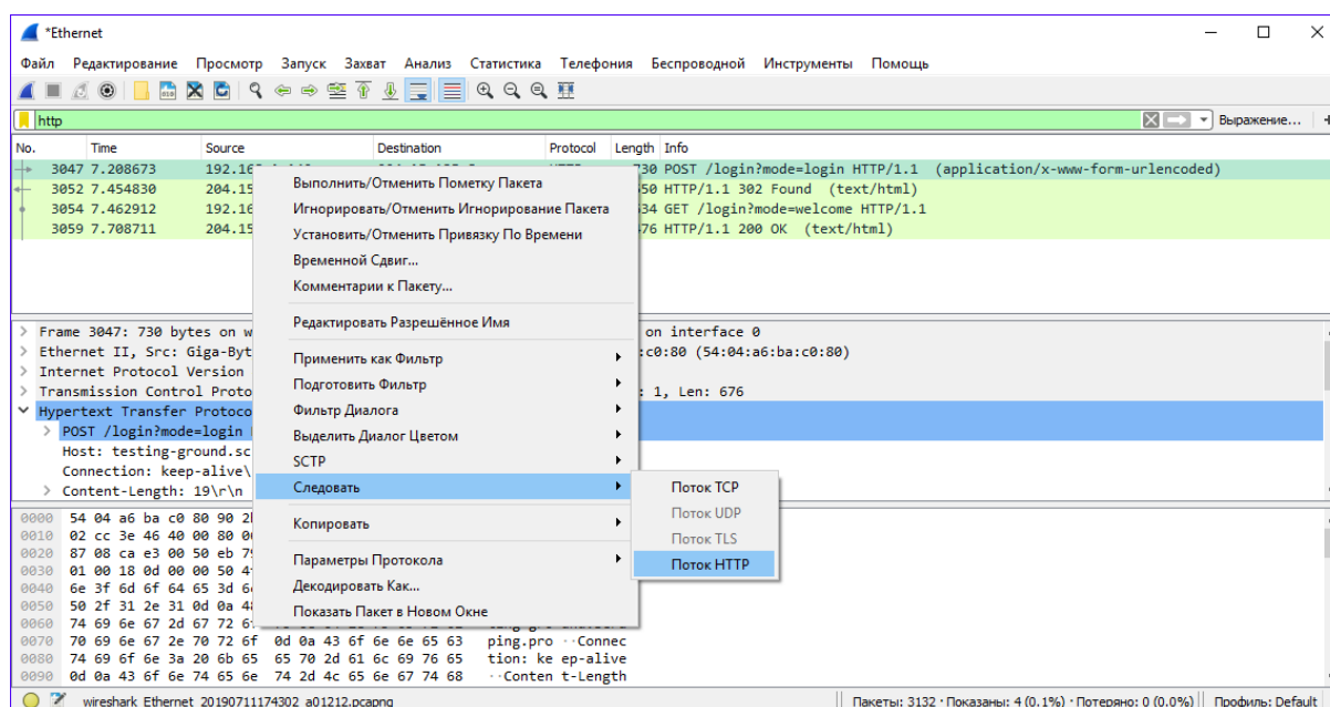
Рисунок 8 – Контекстное меню
