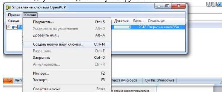
Рис.14 – Создание ключей
