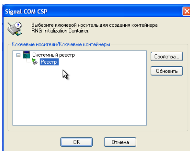
Рисунок 4.9 — Выбор контейнера
