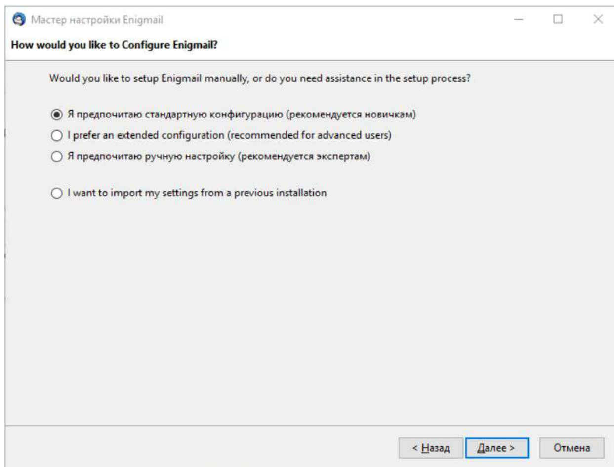
Рис. 7 Выбор конфигурации
