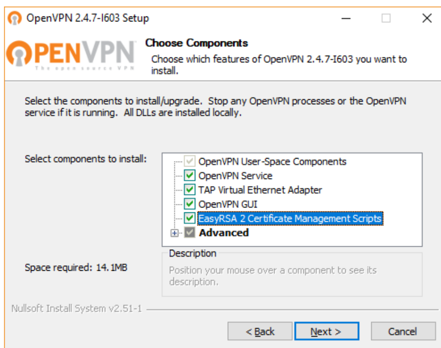
Рисунок 1.5 – EasyRSA
