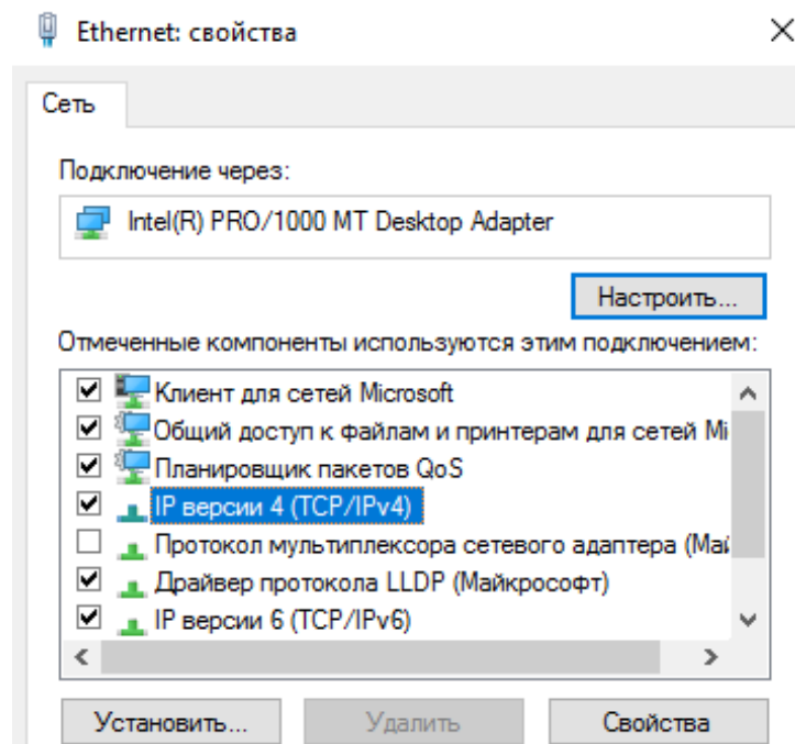
Рис. 4. Ethernet свойства
