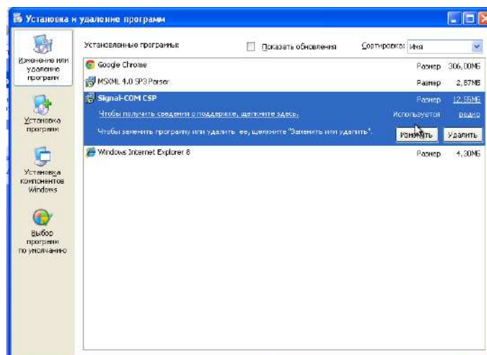
Рисунок 4.7 — Внесение изменений
