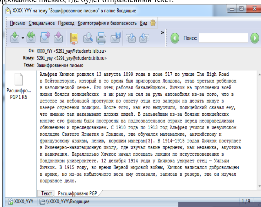
Рис.25 – Расшифрованное сообщение
