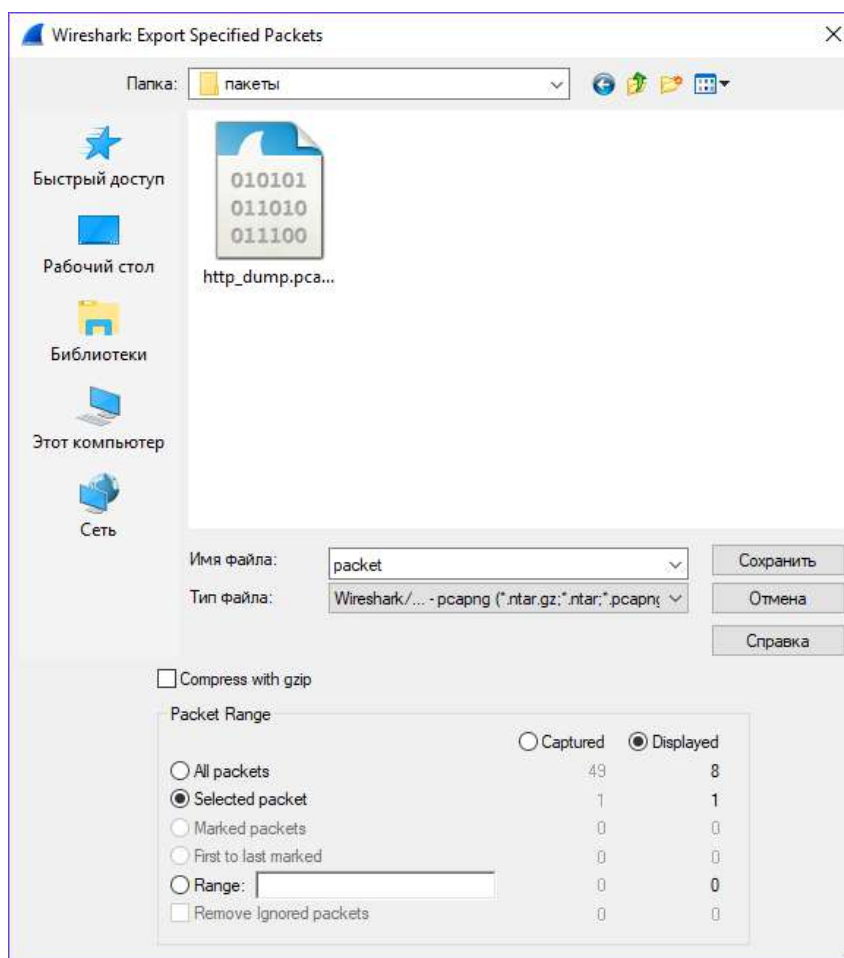
Рисунок 18 – Сохранение пакета
