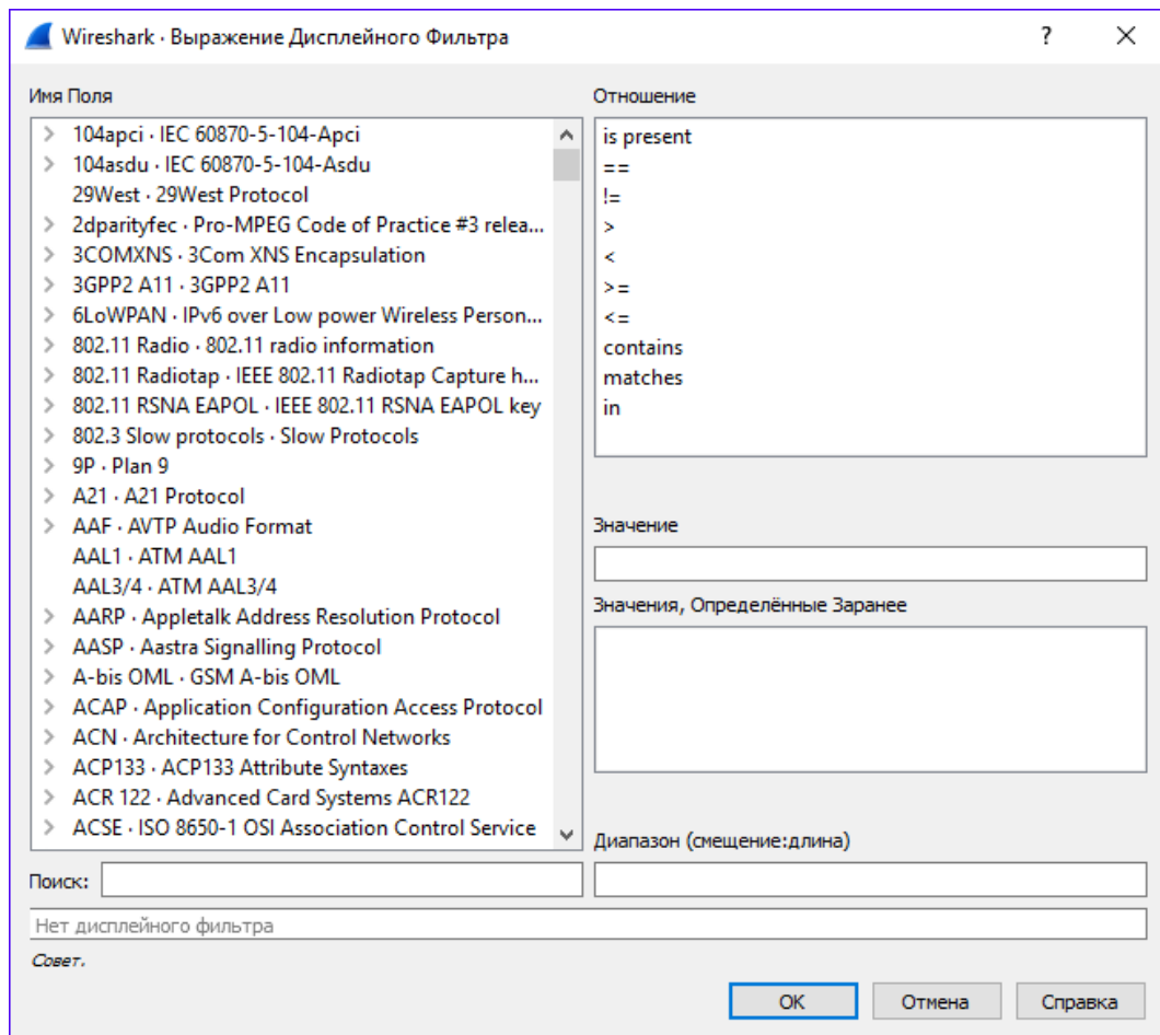
Рисунок 5 – Выражения
