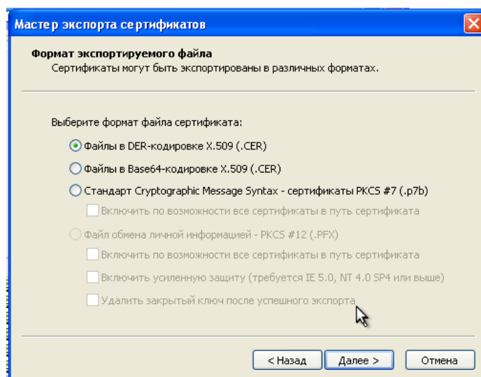
Рисунок 4.22 — Экспорт сертификата
