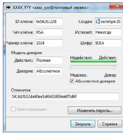
Рис.19 – Свойства ключа
