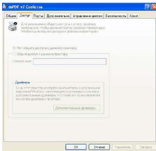
Рисунок 40 – Свойства принтера
