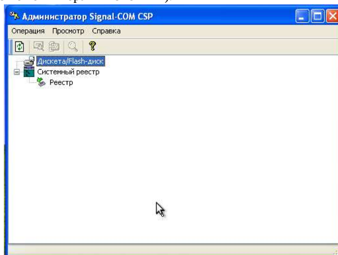
Рисунок 4.6 — Основное окно
