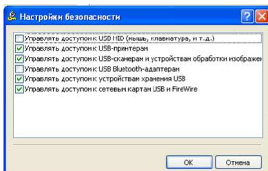
Рисунок 9 – Настройки безопасности
