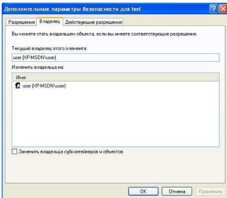
Рисунок 25 – Вкладка «Владелец»
