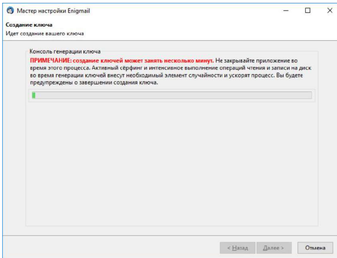
Рис. 10 Создание ключей
