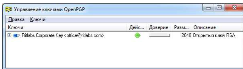
Рис.13 – Библиотека ключей
