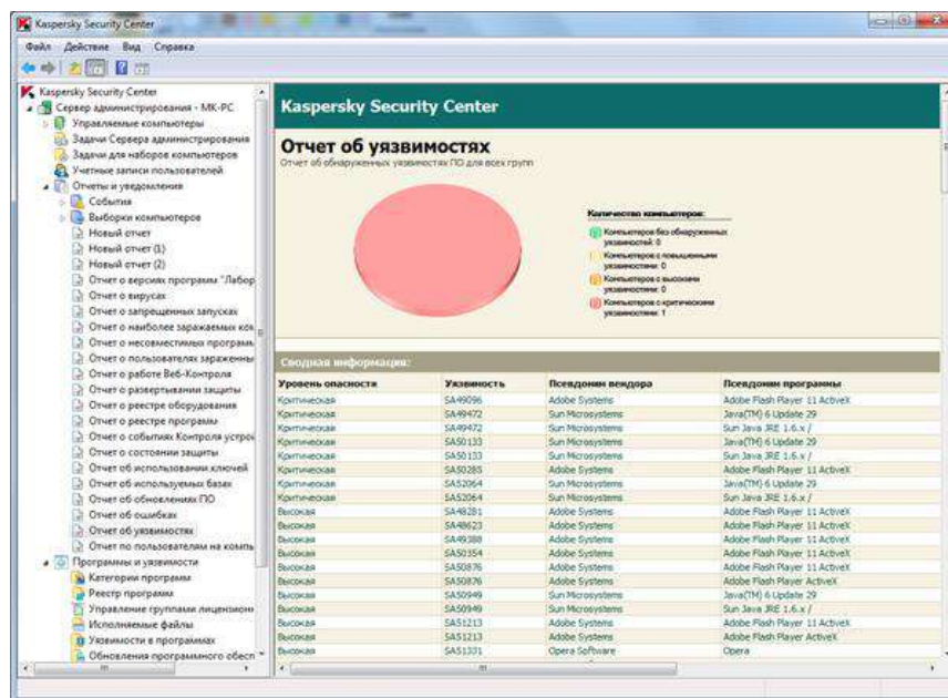
Рисунок 17 – Отчет о поиске уязвимостей.
