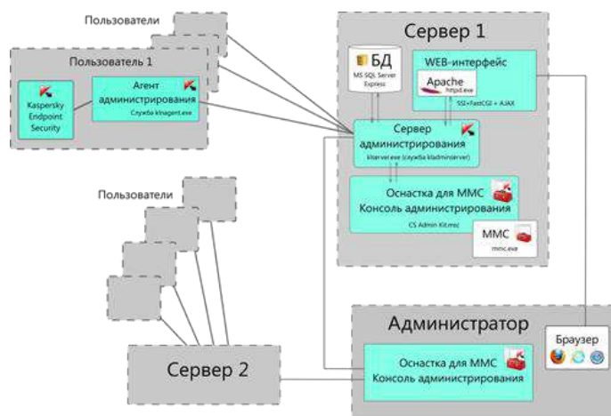
Рисунок 2 – Структурная схема взаимодействия компонентов Kaspersky Security Center.
