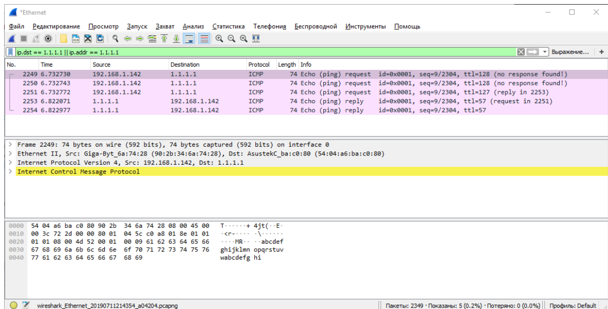
Рисунок 20 – Захваченный сгенерированный пакет
