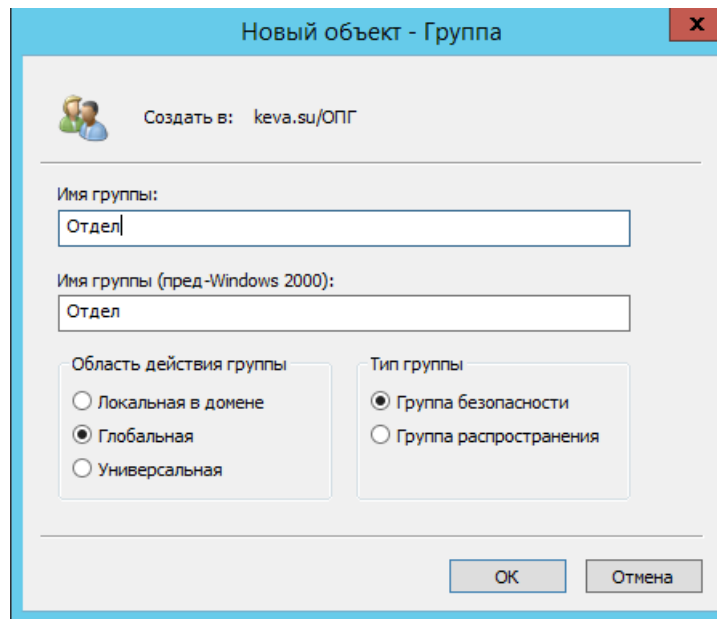
Рис. 13. Создание группы
