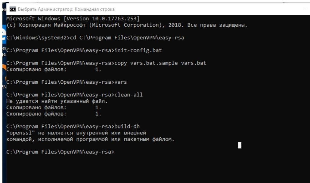
Рисунок 2.4 – Ошибка
