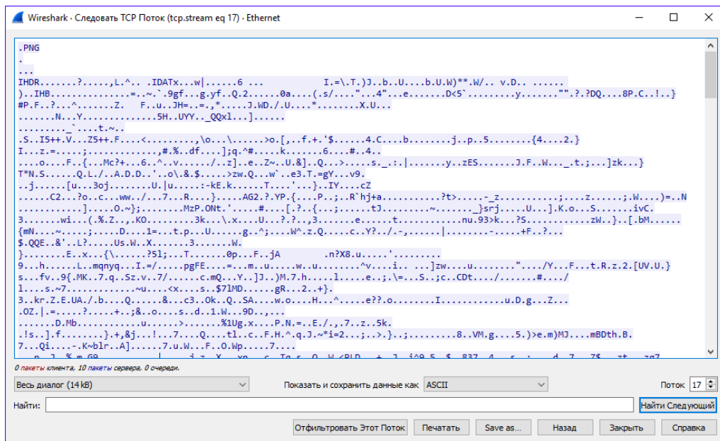
Рисунок 12 – TCP Поток
