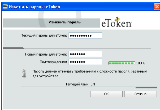
Рисунок 2 – Смена PIN-кода
