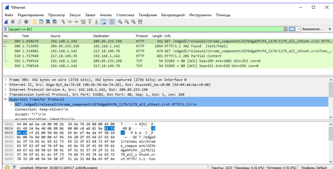
Рисунок 6 – Использование фильтра
