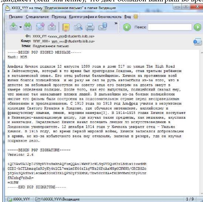
Рис.26 – Подписанное письмо
