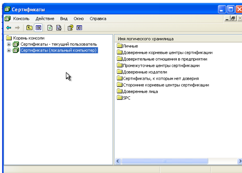
Рисунок 4.19 — оснастка сертификатов
