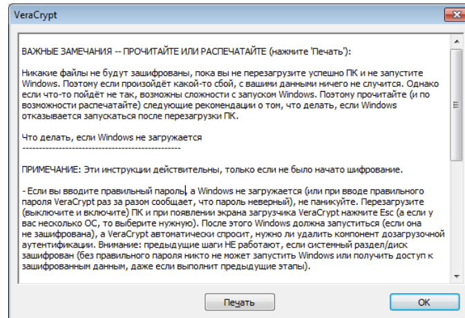
Рисунок 51 – Информационное сообщение
