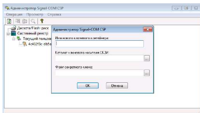
Рисунок 4.10 – Импорт сертификата
