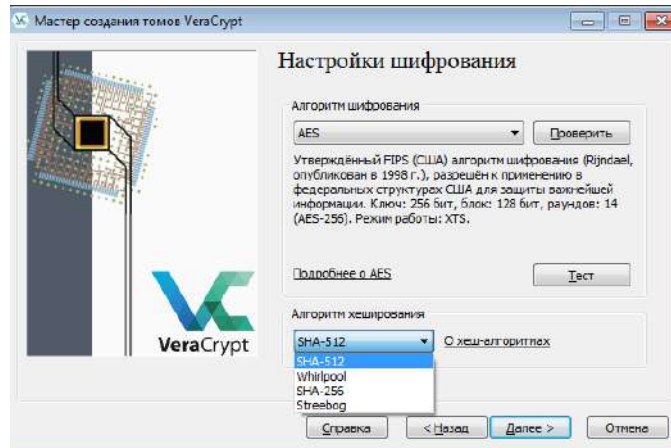
Рисунок 8 – Алгоритмы хеширования
