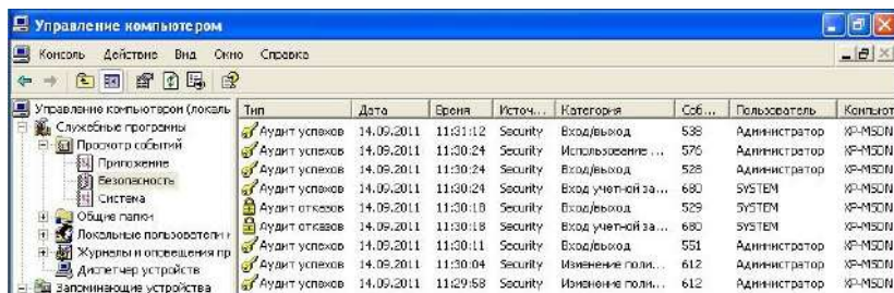
Рисунок 3 – Журнал «Безопасность»
