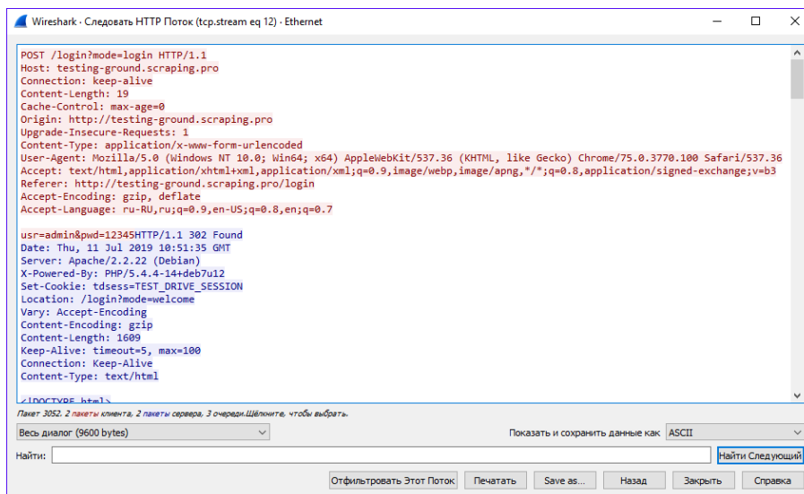
Рисунок 9 – HTTP Поток
