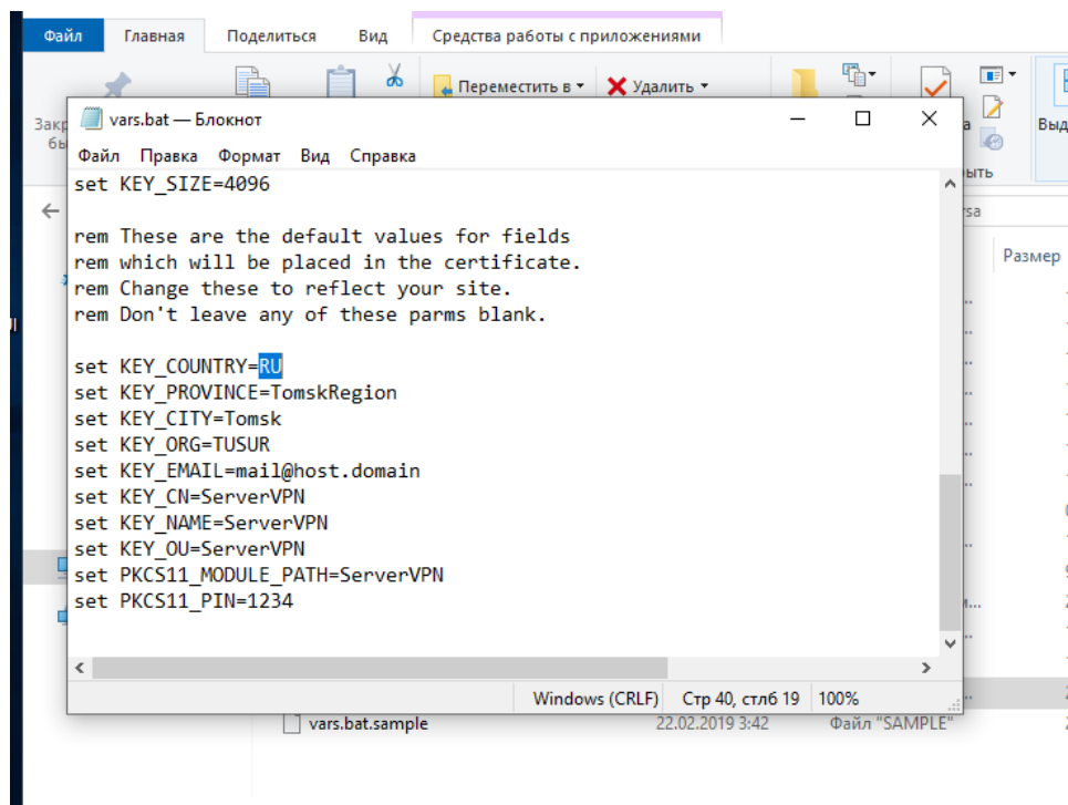
Рисунок 2.2 – vars.bat
