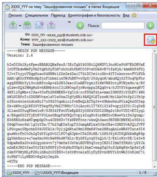
Рис.24 – Зашифрованное письмо
