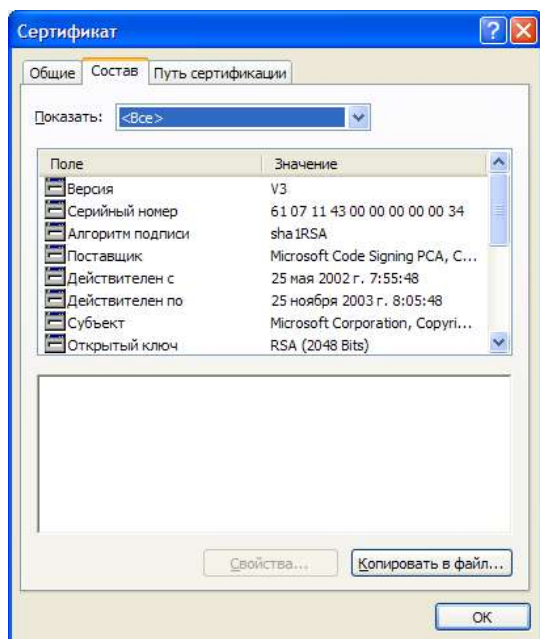
Рисунок 12 – Сертификат
