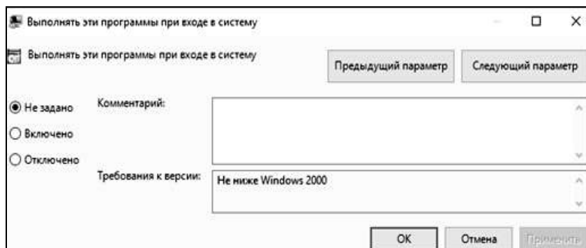
Рис. 38. Включение параметра
