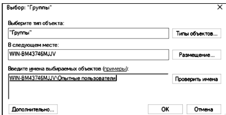
Рис. 13. Добавление группы
