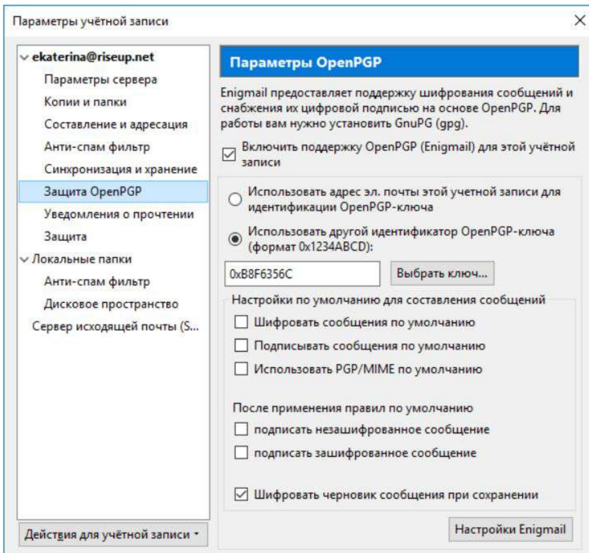
Рис. 18 Параметры OpenPGP
