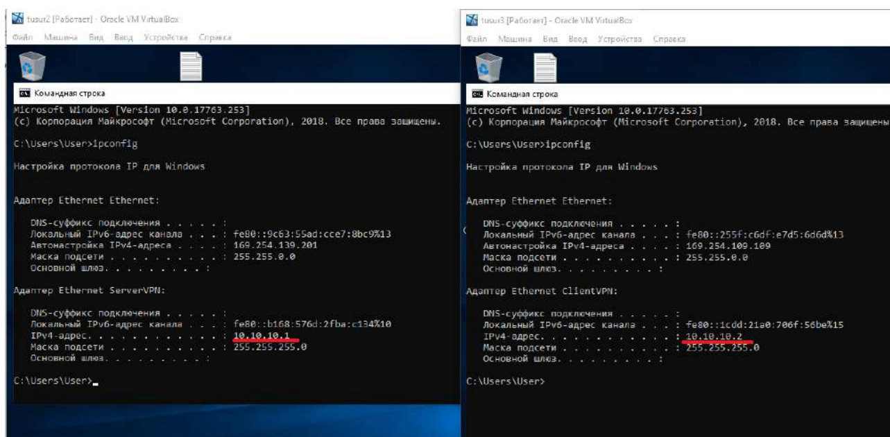
Рисунок 4.8 – Проверка ip
