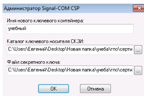
Рисунок 4.11 – Настройка импорта
