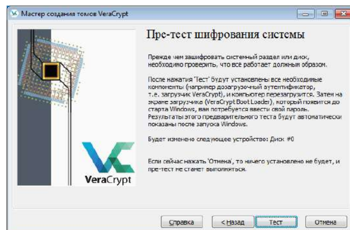
Рисунок 49 – Пре-тест
