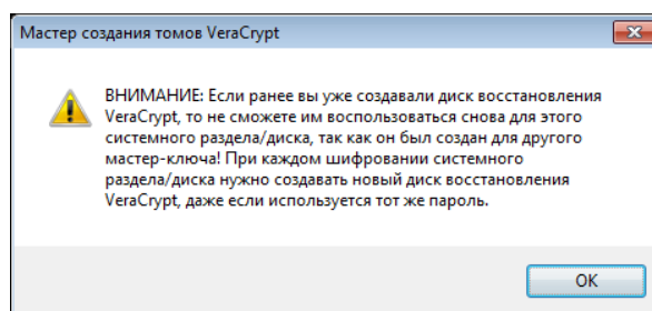
Рисунок 47 – Предупреждение
