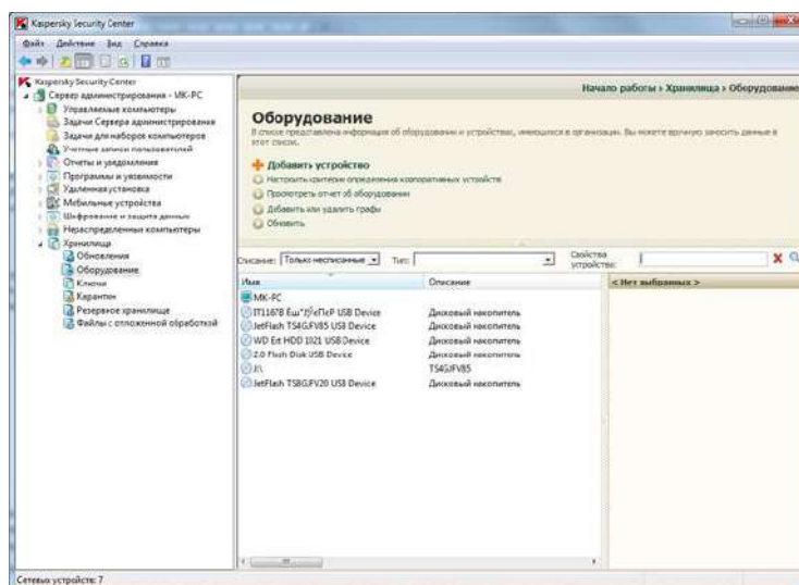
Рисунок 12 – Хранилище оборудования.
