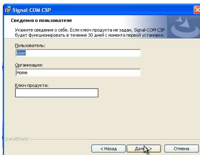
Рисунок 4.2 — Ввод ключа
