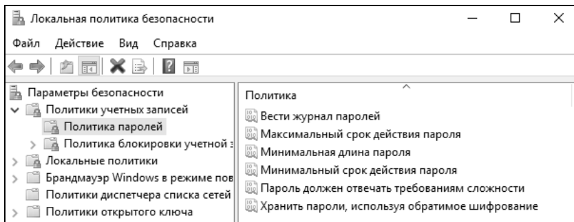
Рис. 28. Политика паролей
