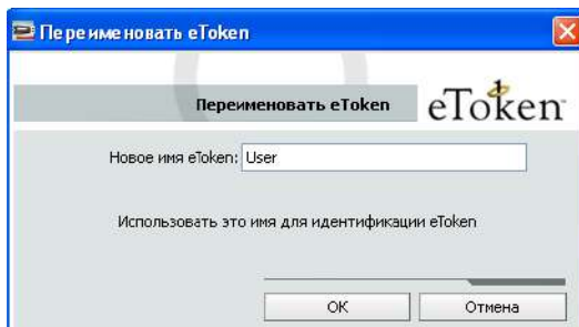
Рисунок 3 – Переименование eToken
