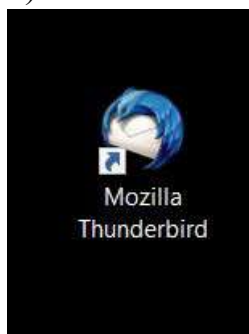
Рис. 1 Mozilla thunderbird
