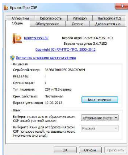
Рисунок 4.18 – КриптоПро CSP
