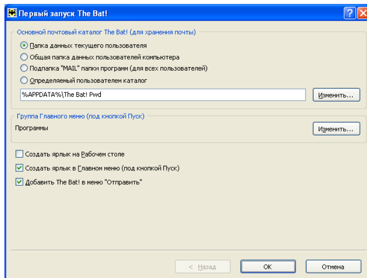
Рис.2 – Первый запуск
