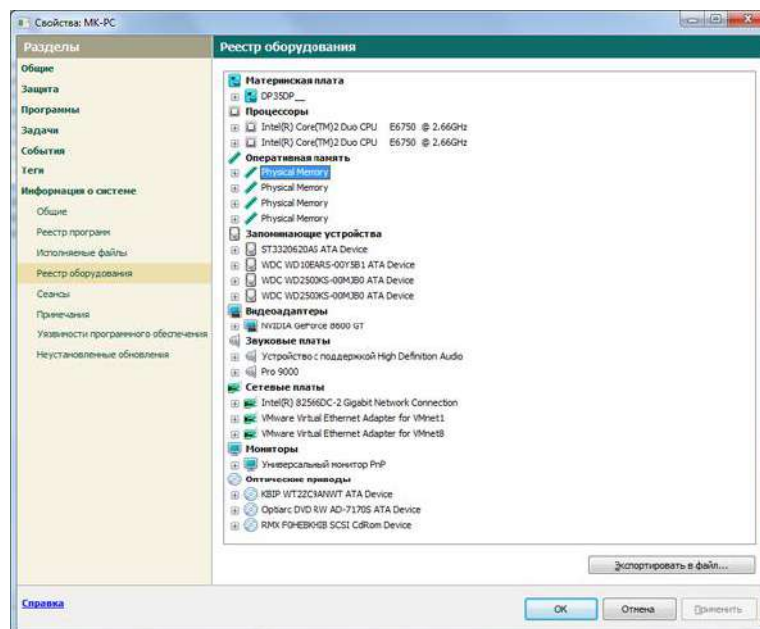
Рисунок 13 – Реестр оборудования.
