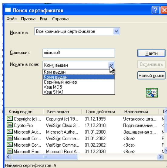
Рисунок 4.20 — Поиск сертификатов.
