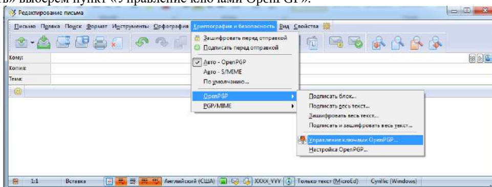
Рис.12 – Выбор пункта
