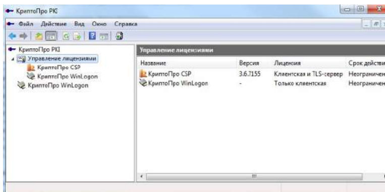
Рисунок 4.17 – КриптоПро PKI
