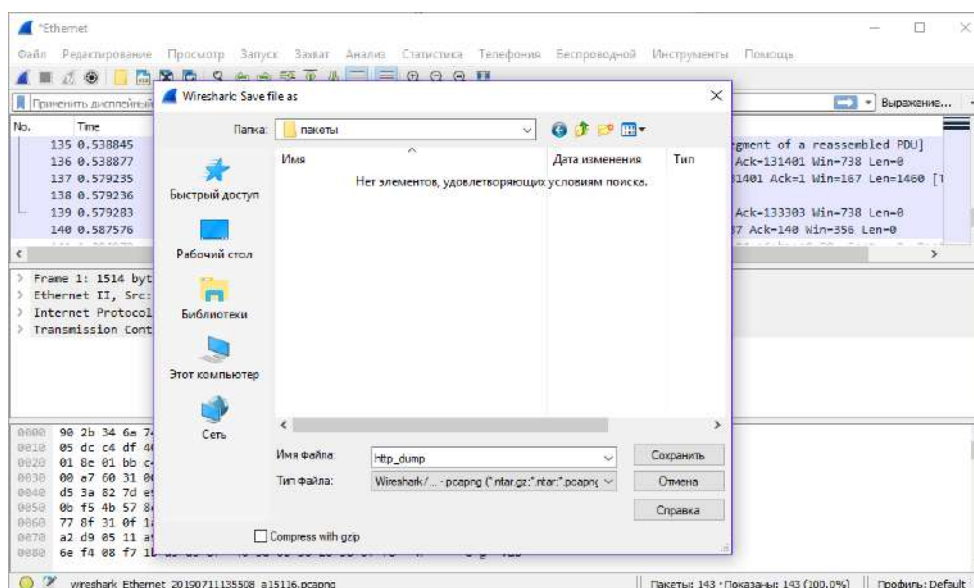
Рисунок 7 – Сохранение дампа
