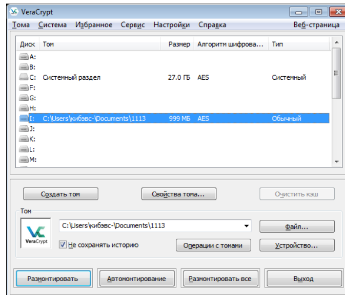
Рисунок 18 – Смонтированный раздел
