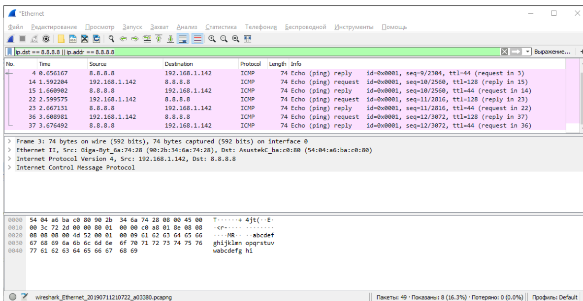
Рисунок 16 – Найденные пакеты
