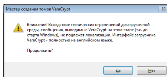
Рисунок 50 – Предупреждение
