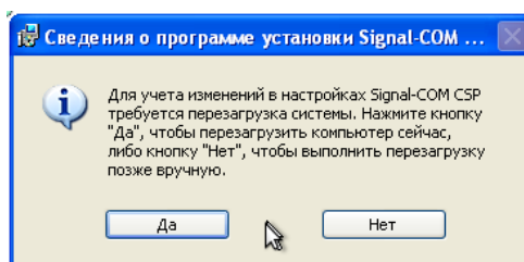
Рисунок 4.4 — Завершение установки
