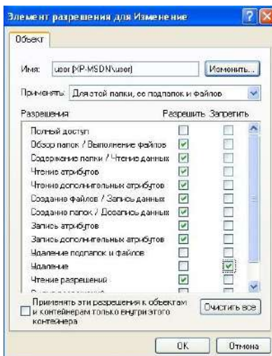
Рисунок 21 – Запрет удаления
