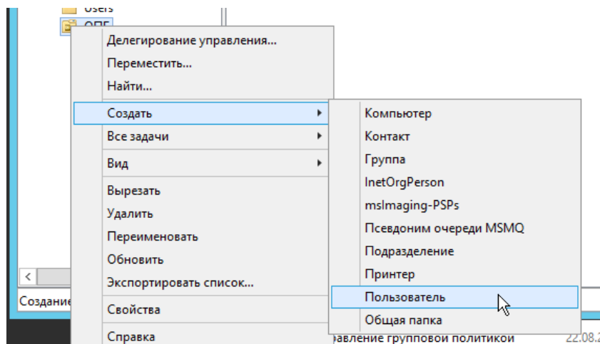
Рис. 11. Контекстное меню
