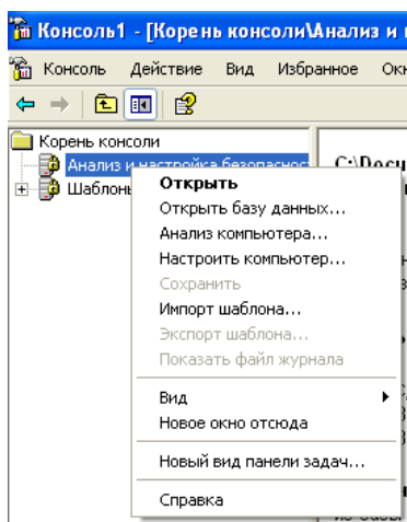
Рисунок 15 – Импорт шаблона
